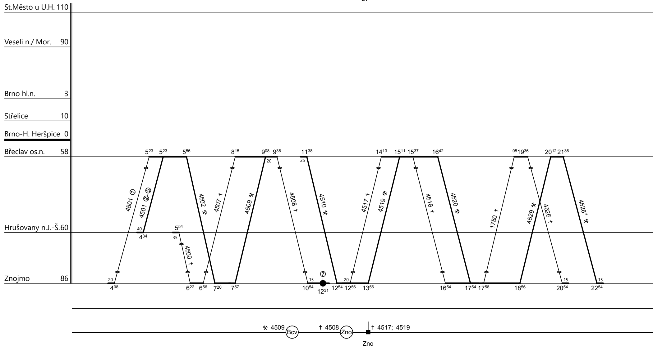
Výkony 3. TD veze TS 8271 PP Znojmo
